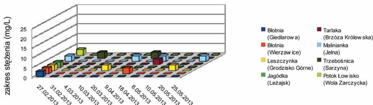
Wykres 2. Zależność stężenia fosforanów (V) od czasu badania w rzekach powiatu leżajskiego.
